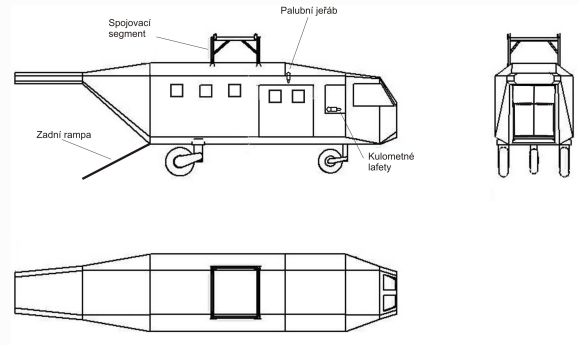
Schéma závěsného vysazovacího modulu.
