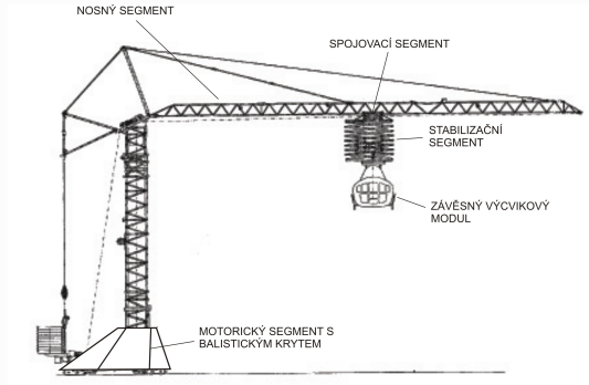
Přehledové schéma trenažéru.
