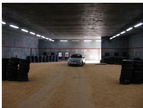
Zónová balistická ochrana rozdělená na zónu vysokého zatížení střelbou a zónu zachytávání náhodných výstřelů.
