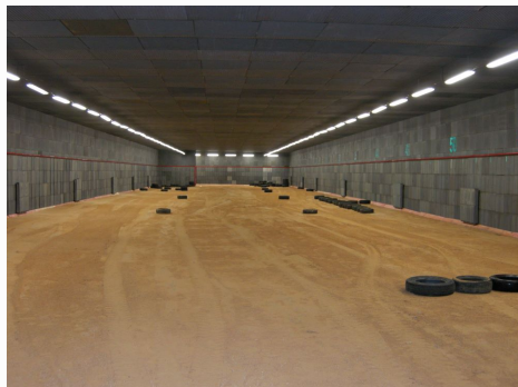
Pohled na balistickou ochranu stěn střelnice dlouhé 82 m.
