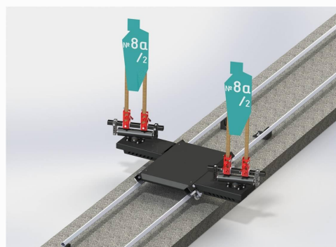
Dálkově ovládaný pojízdný vozík na umístění různých terčových zvedáků.
